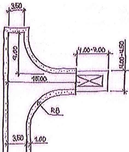
Bild 2. Exempel på uppställningsplats för container
