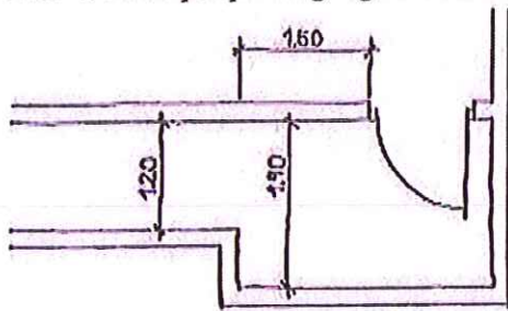
Bild 4. Exempel på dragvägs bredd vid riktningsändring 1
