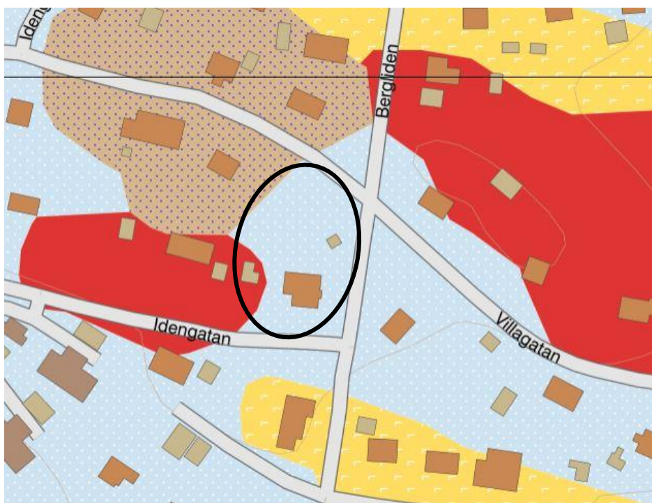
Jordartskarta från SGU ( www.sgu.se ), planområdet markerat med svart ring.
